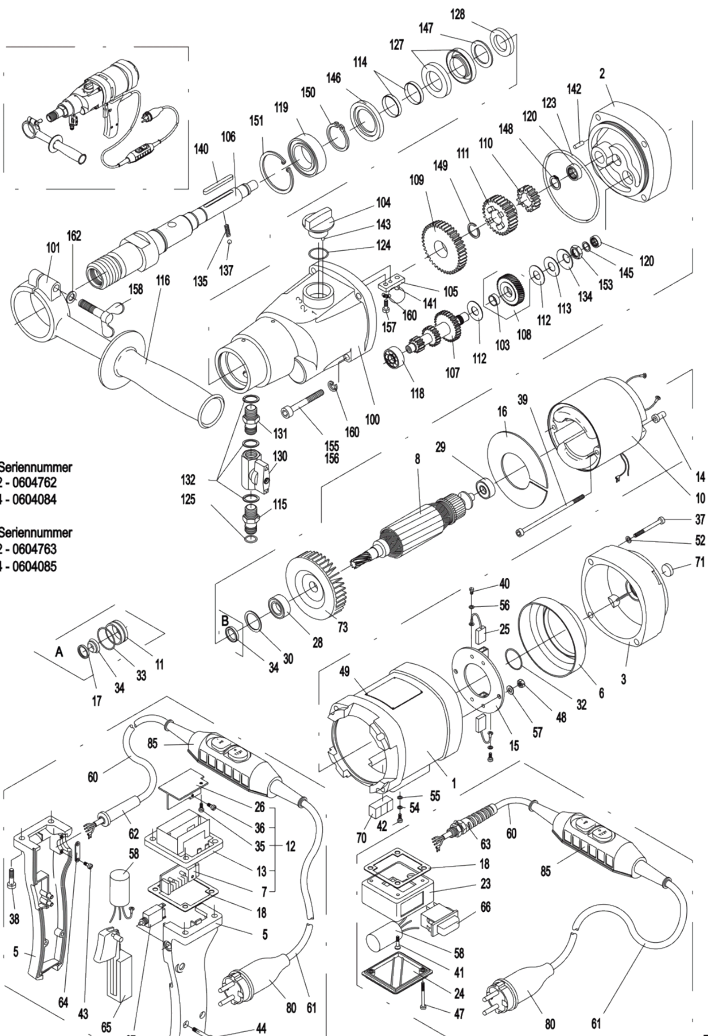
TYP DK 12/16
